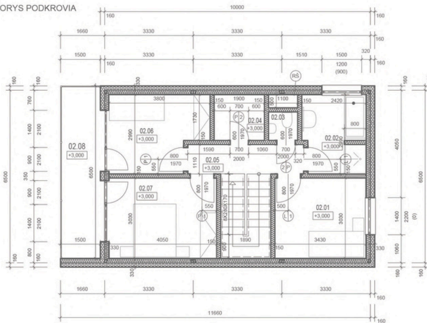
PODORYS PODKROVIA
